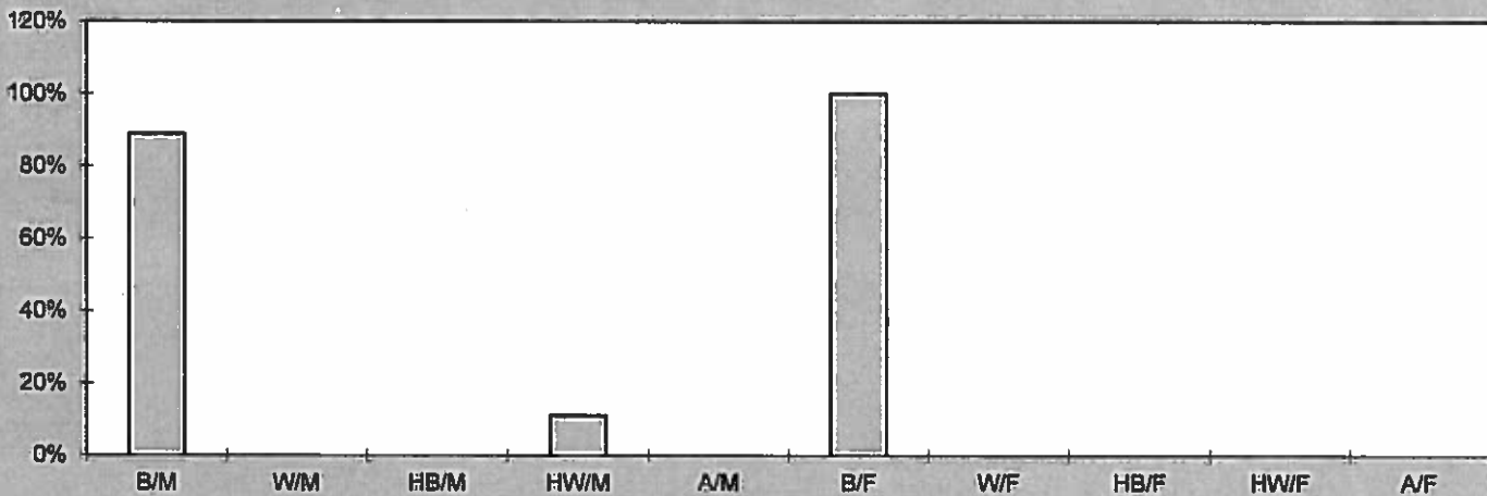
VICTIM %
